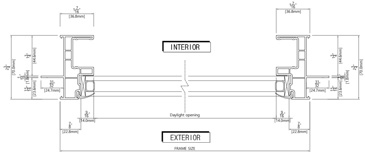
3 B-B' SECTION JAMB
